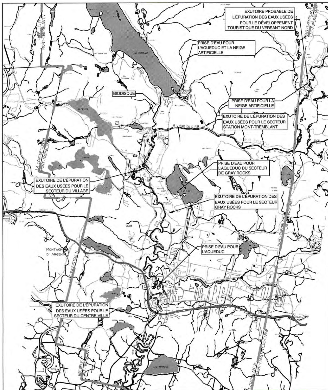
Figure 3 – Prises d'eau et exutoires
